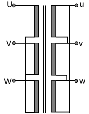
●結線図
